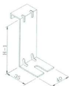
外側固定片
