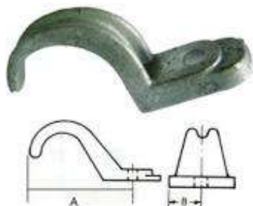
單孔管夾 MW
